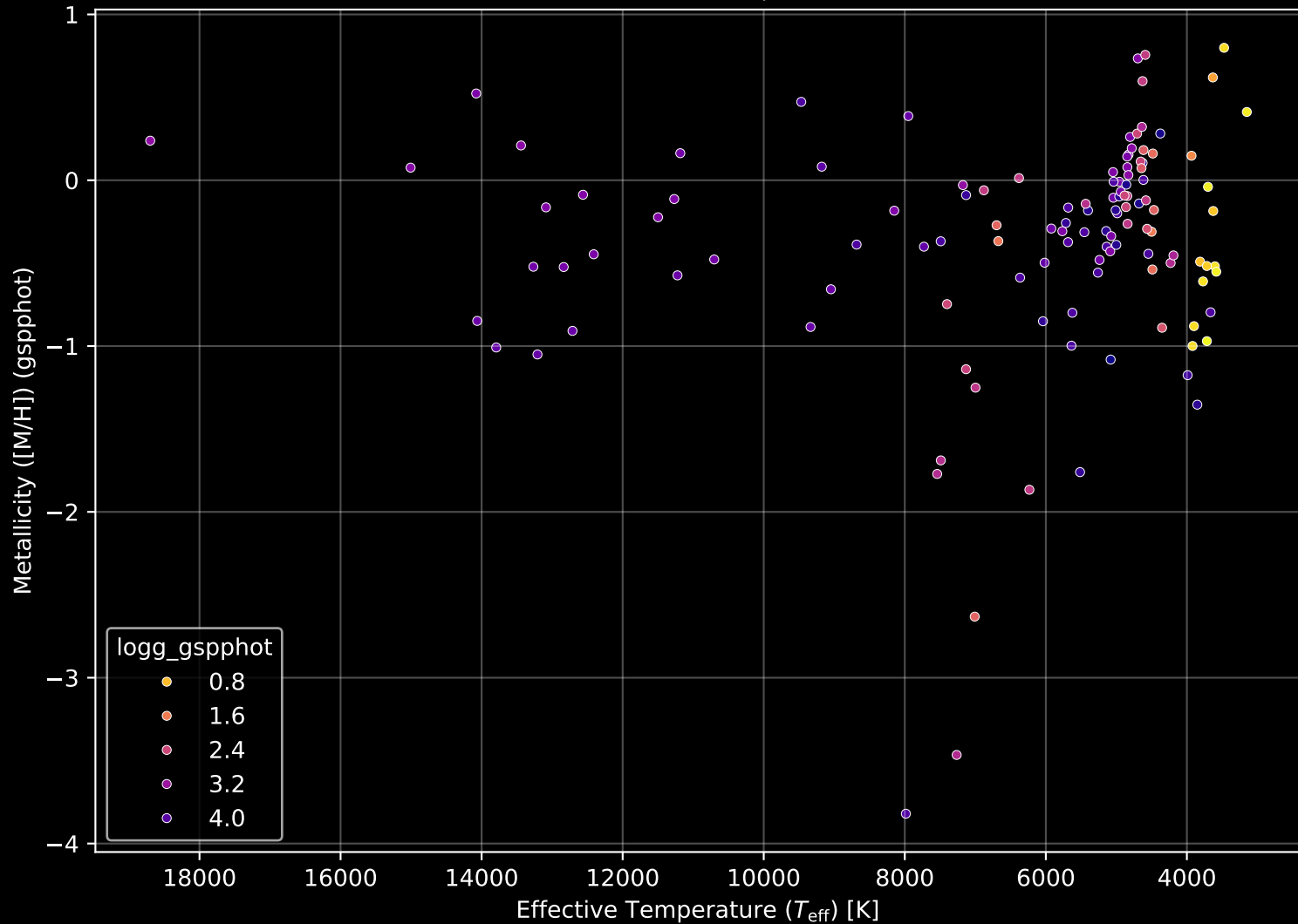
APOGEE DR17 Field: [014+00] Stellar Population Parameters (n= 122)
